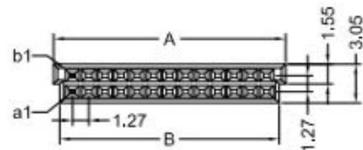
- Interface Dim. -
