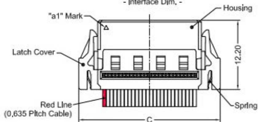
- Interface Dim. -
